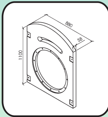
• Pro Panel
