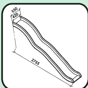
• Long Slide
