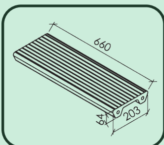
• Step
