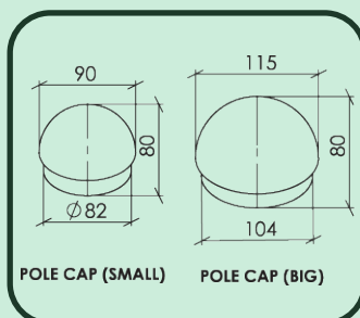
• Pole Cap
